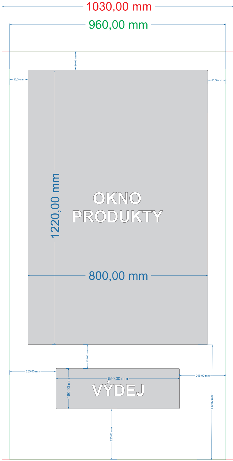
PŘEDNÍ ČÁST „1“ AUTOMATU výška 1810mm x šířka 960mm tiskový rozměr výška 1810mm x šířka 1030mm samolepka s přelepem
