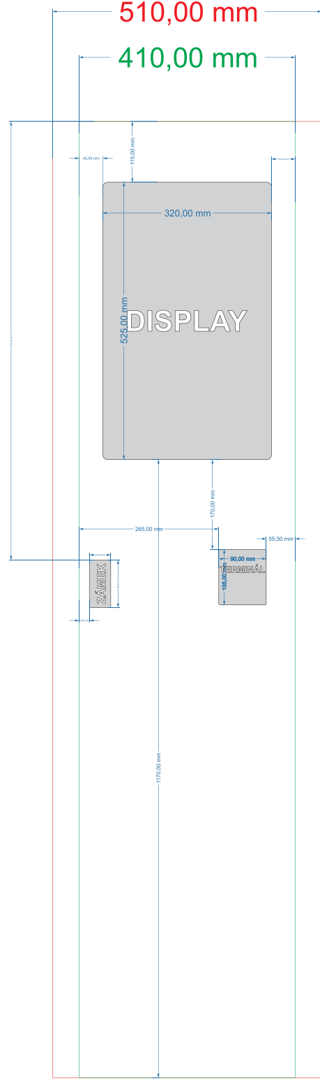
PŘEDNÍ ČÁST „2“ AUTOMATU výška 1810mm x šířka 410mm tiskový rozměr výška 1810mm x šířka 510mm samolepka s přelepem
